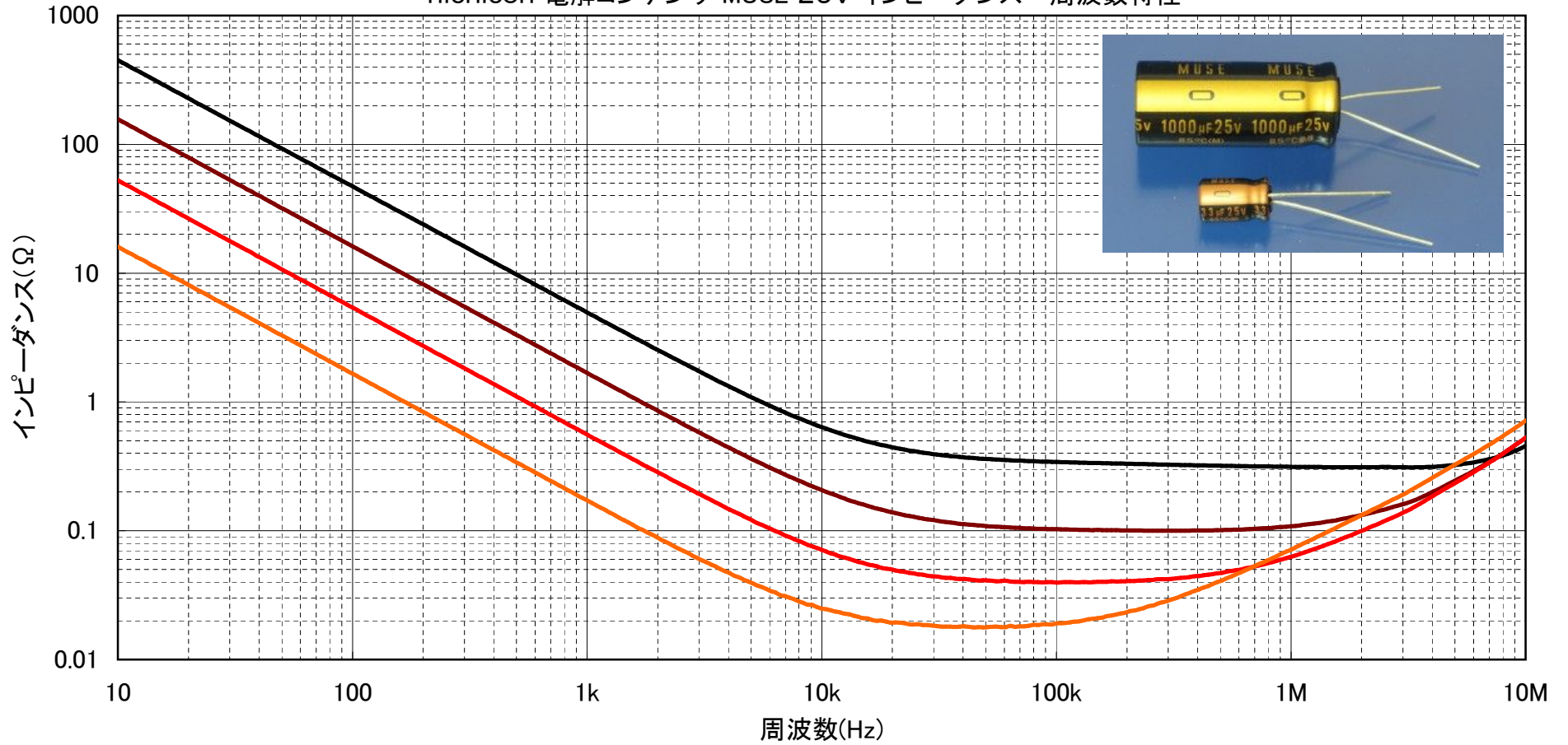
nichicon 電解コンデンサ MUSE 25V インピーダンス-周波数特性
