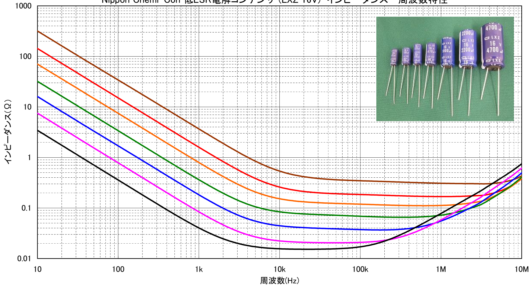
Nippon Chemi-Con 低ESR電解コンデンサ (LXZ 16V) インピーダンス-周波数特性
