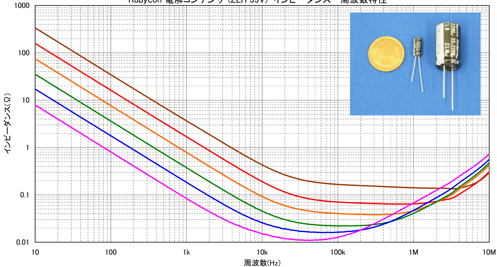
Rubycon 電解コンデンサ (ZLH 35V) インピーダンス-周波数特性
