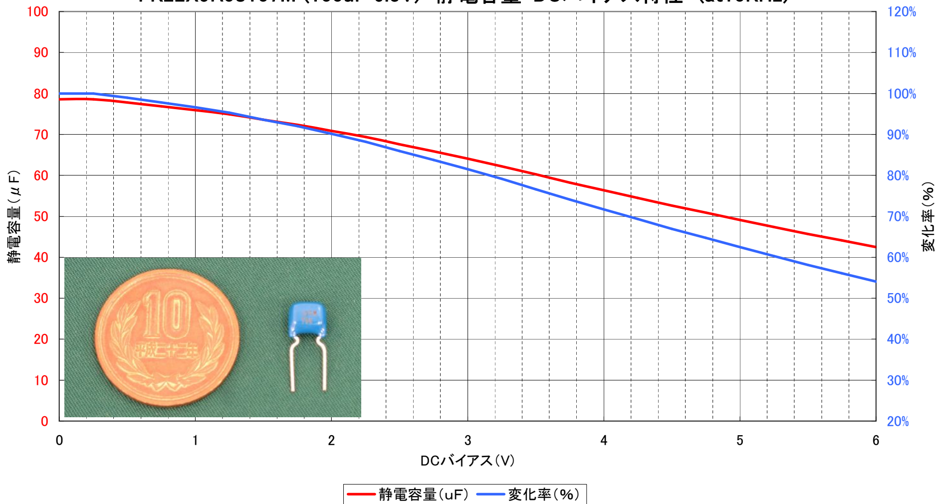
FK22X5R0J107M (100uF 6.3V) 静電容量-DCバイアス特性 (at10KHz)
