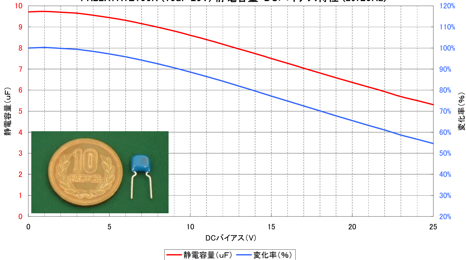
FK22X7R1E106K (10 \mu F 25V) 静電容量-DCバイアス特性 (at120Hz)
