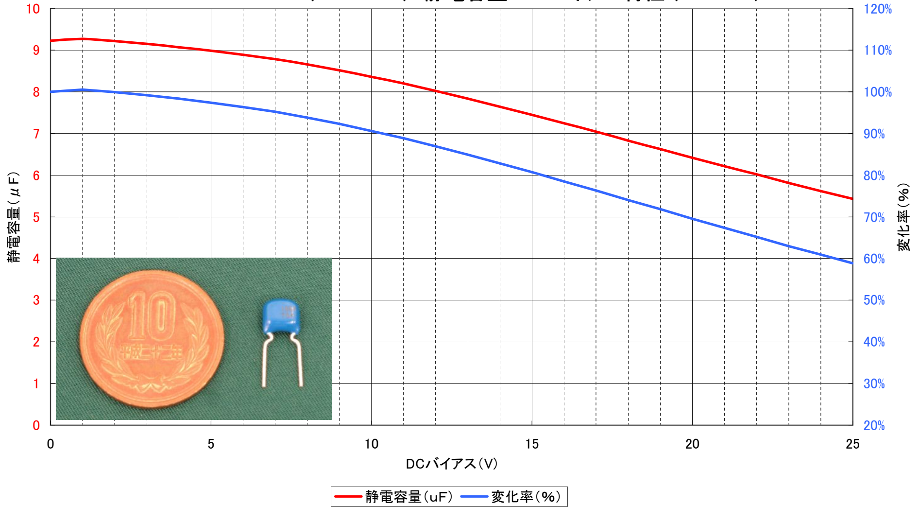
FK22X7R1E106K (10 \mu F 25V) 静電容量-DCバイアス特性 (at10KHz)
