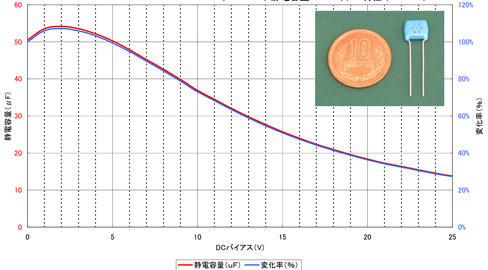
NIPPON CHEMI-CON THD41E1E476Z (47 \mu F 25V) 静電容量-DCバイアス特性 (at10KHz)
