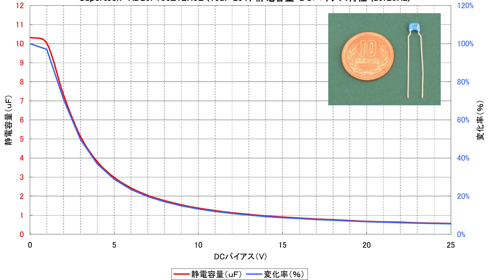
Supertech RD20F106Z1EH5L (10uF 25V) 静電容量-DCバイアス特性 (at120Hz)
