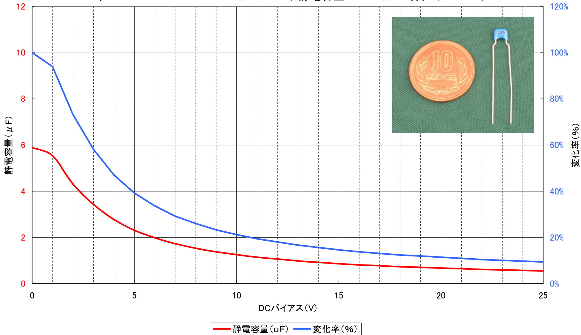
Supertech RD20F106Z1EH5L (10uF 25V) 静電容量-DCバイアス特性 (at10KHz)
