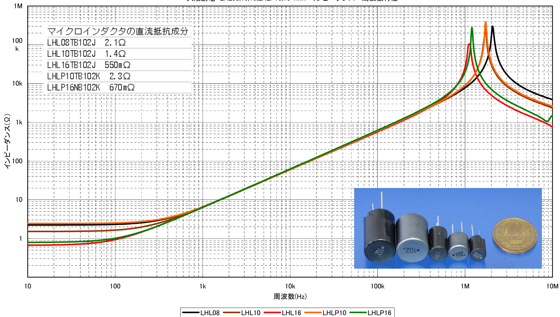
大陽誘電 LHL08,10,16,LHLP10,16 1mH インピーダンス-周波数特性
