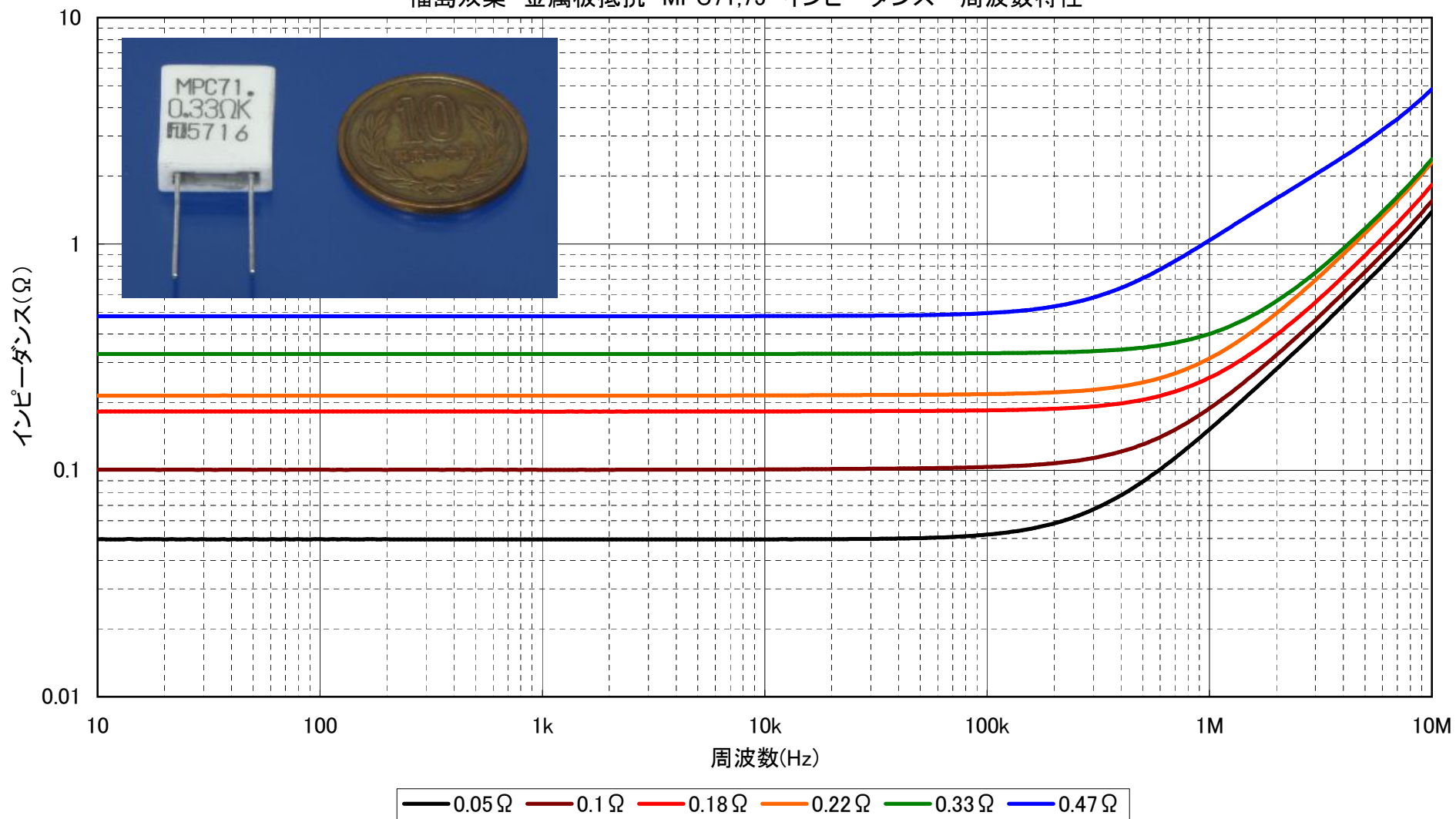
福島双葉 金属板抵抗 MPC71,75 インピーダンス-周波数特性
