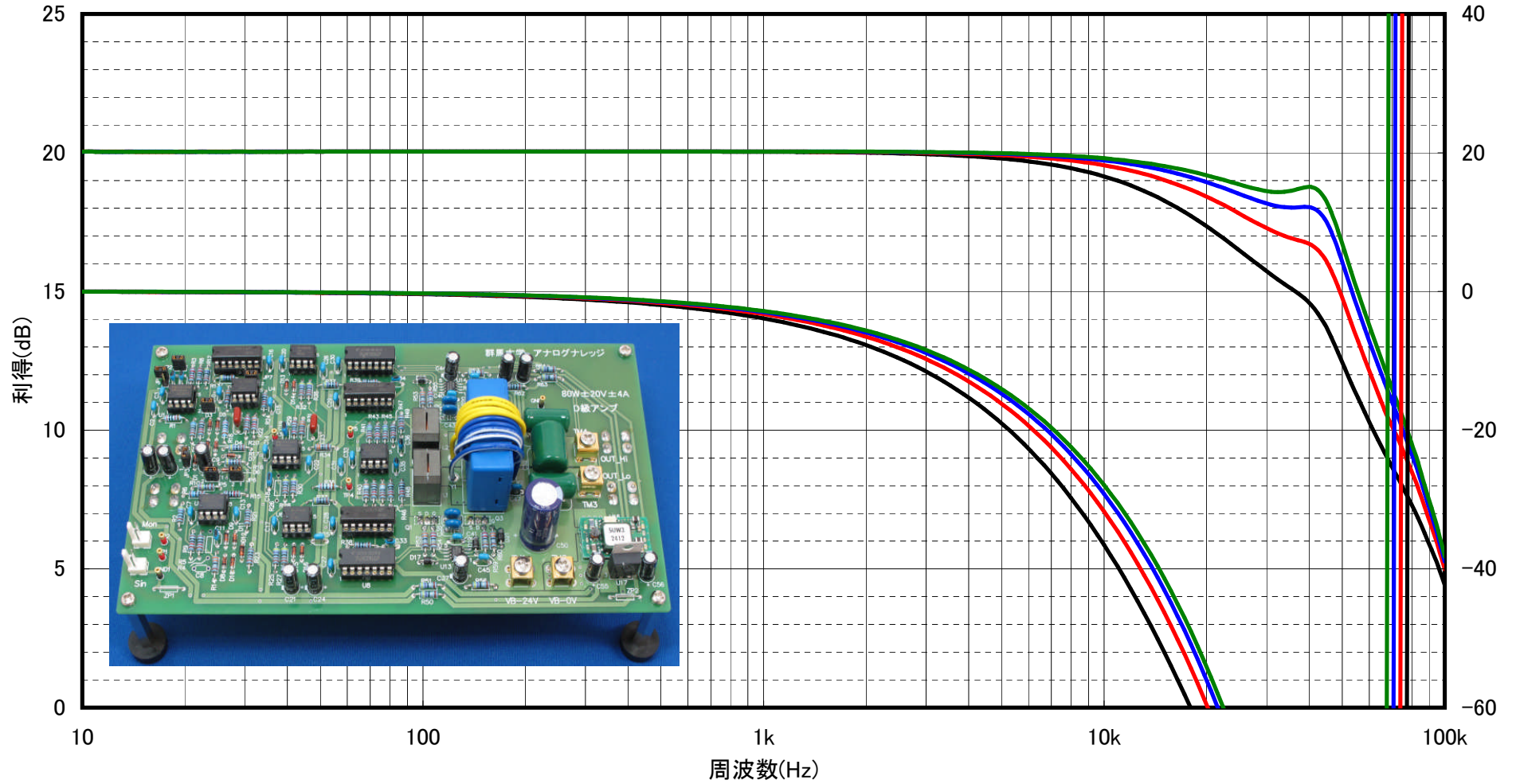
ナレッジ・パワエレクトロニクスセミナ用D級アンプ周波数特性
